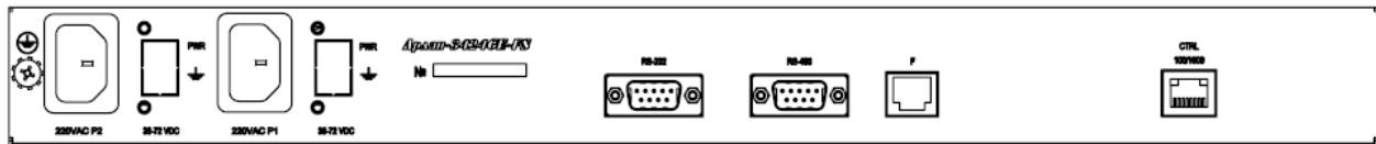
Рисунок Б.2 – Внешний вид задней панели коммутатора
