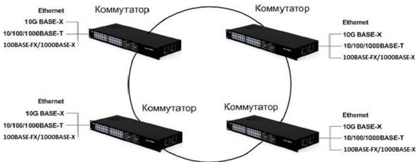
Рисунок 2 – Включение коммутаторов в кольцевую топологию
